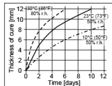
Diagram 1: Rýchlosť vytvrdzovania Sikaflex®-252
