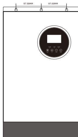
Terminal (wymiary)
