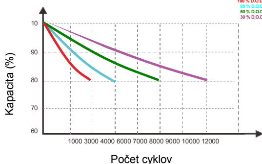
Různé DOD Životnost' vybíjecího cyklu Krivka 0,2C 25 °C
