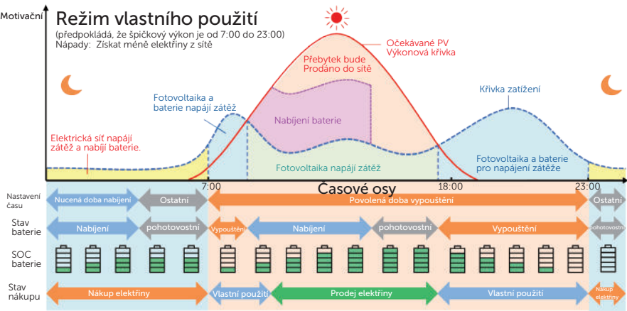
Obrázky- 210 Režim vlastního použití
