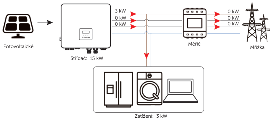
Obrázky- 216 Povolit ovládání nulového výstupu pro fázovou nerovnováhu
