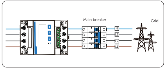
Obrázky- 1528 Připojení přímého měřiče k elektrické síti
