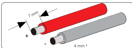
Obrázky- 822 Odstraňování fotovoltaických kabelů
