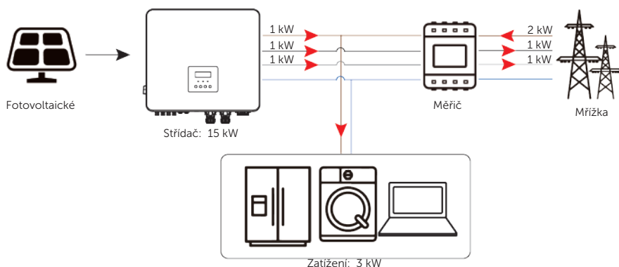
Obrázky- 215 Zakázat ovládání nulového exportu pro fázovou nerovnováhu
