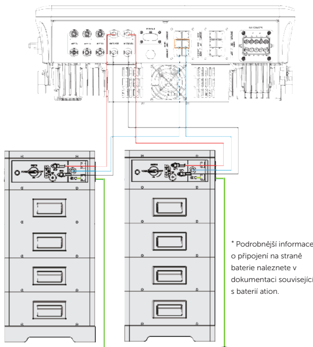
Obrázky- 845 Schéma připojení BMS
