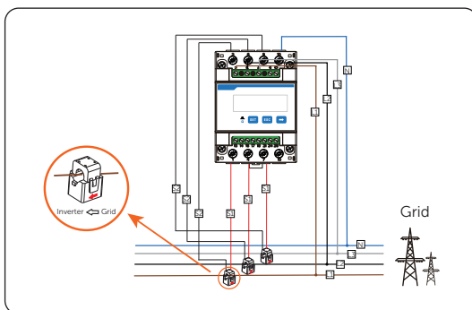
Obrazky- 1532 Připojení CT připojených měřičů k elektrické síti
