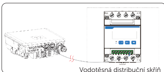
Obrázky- 1534 Připojení střídače k měřiči
