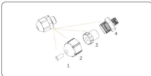
Obrázky- 863 Odstraňte vodotěsný konektor
