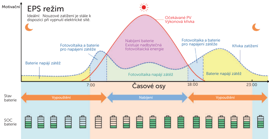
Obrázky- 214 EPS režim
