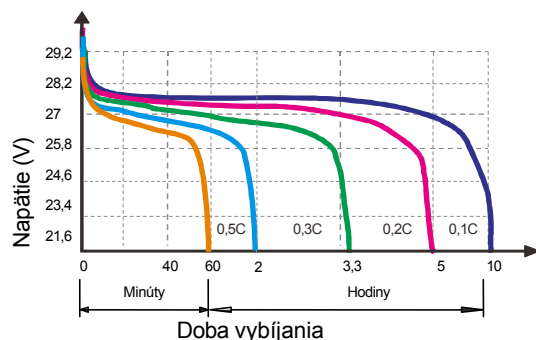
Vybíjacie charakteristiky pri 25 °C
