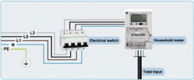
Trójfazowy 400 V
