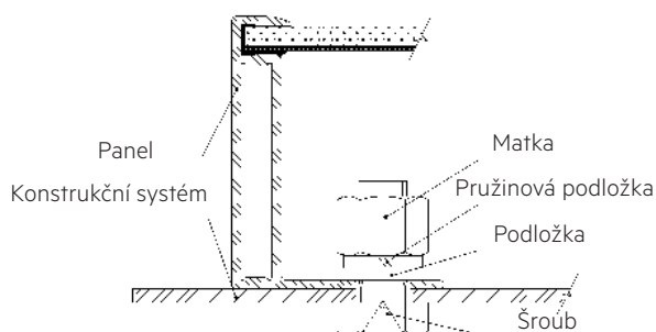
Obrázek 3: Příklad šroubování
