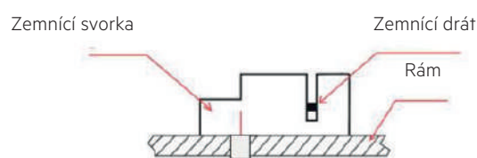
Obr. 7B Zemnicí svorka
